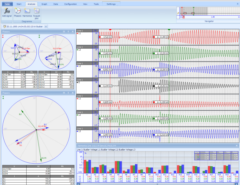
Abb 6: Analyse einer Störfallaufzeichnung
