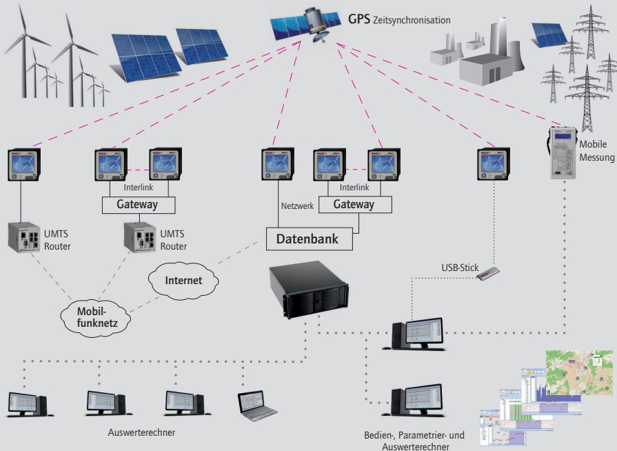
Abb. 3: Kommunikations- und Zeitsynchronisationsmodell
